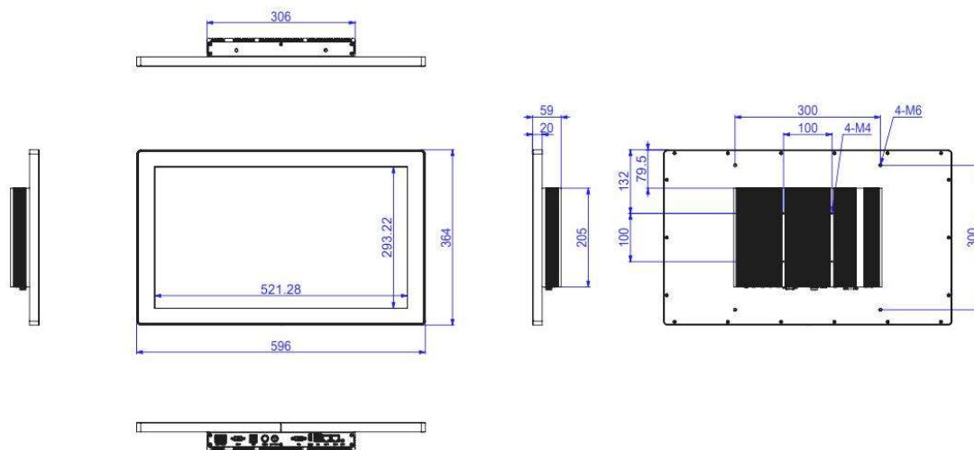
i5-6200U 电容触摸尺寸图
