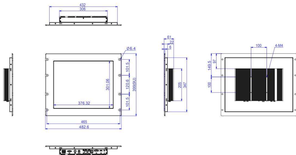
J1900 电阻触摸尺寸图
