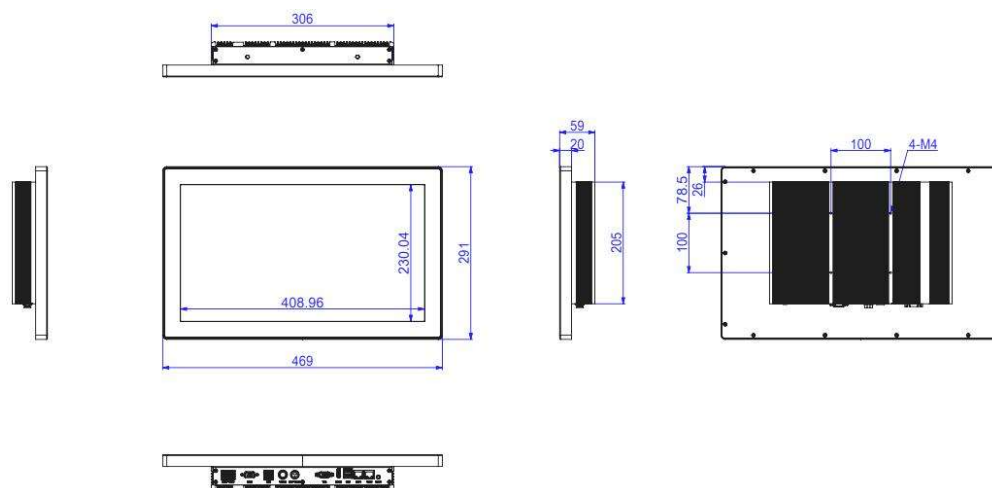
i5-6200U 电容触摸尺寸图
